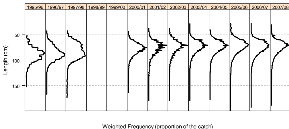
Figure 3 : Fréquences de longueurs pondérées selon la capture pour Dissostichus eleginoides capturé à la palangre dans la ZEE française de la division 58.5.1 (sources : données à échelle précise et données STATLANT ; les relations longueur-poids proviennent des observations de D. eleginoides dans la division 58.5.2).
