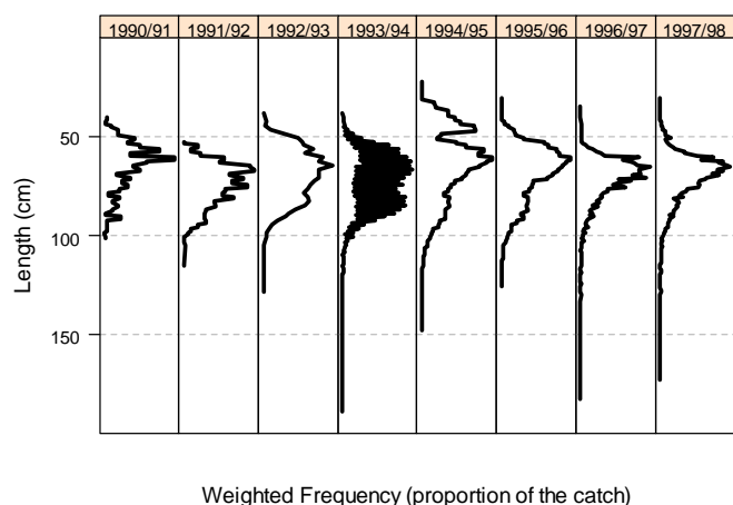
Figure 2 : Fréquences de longueurs pondérées selon la capture pour Dissostichus eleginoides capturé par chalutage dans la ZEE française de la division 58.5.1 (sources : données à échelle précise et données STATLANT ; les relations longueur-poids proviennent des observations de D. eleginoides dans la division 58.5.2).
